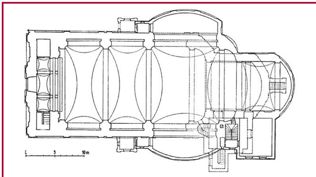
3. kép. Krisztinavárosi Havas Boldogasszony-templom alaprajza (T. M.)
